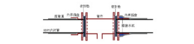
图3 承插连接示意图
