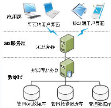
图1 供水管网智能化抢修系统体系结构
