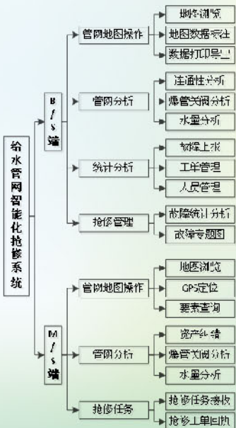
图3 供水管网智能化抢修系统功能框架
